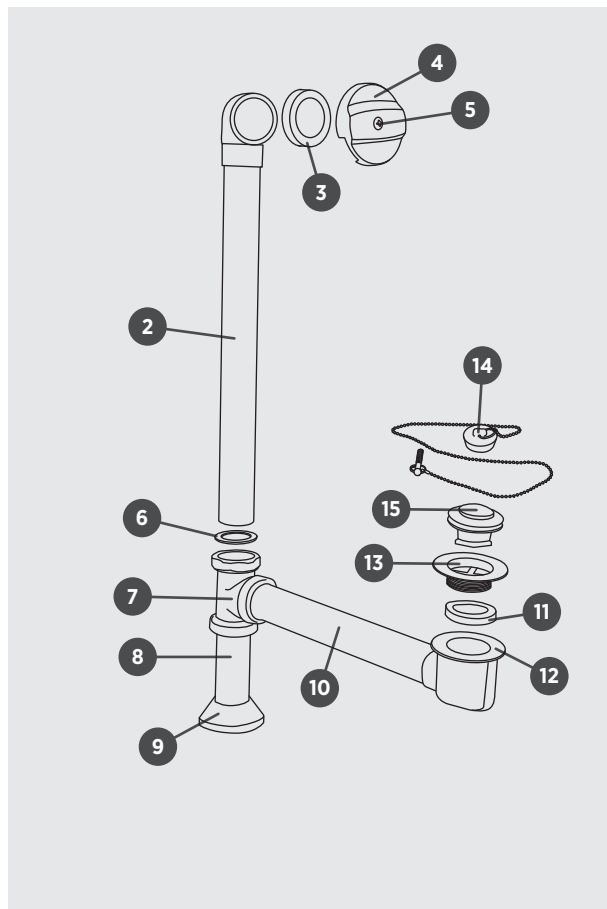
1 | PB-21071-PART D ADAPTER ADAPTATEUR
