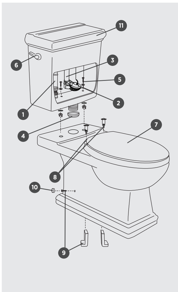
1A | PB-FILLV-H-A2002 FILL VALVE ROBINET DE REMPLISSAGE
